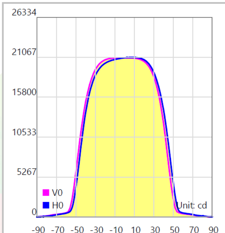
DIAGRAMA CARTESIANO
