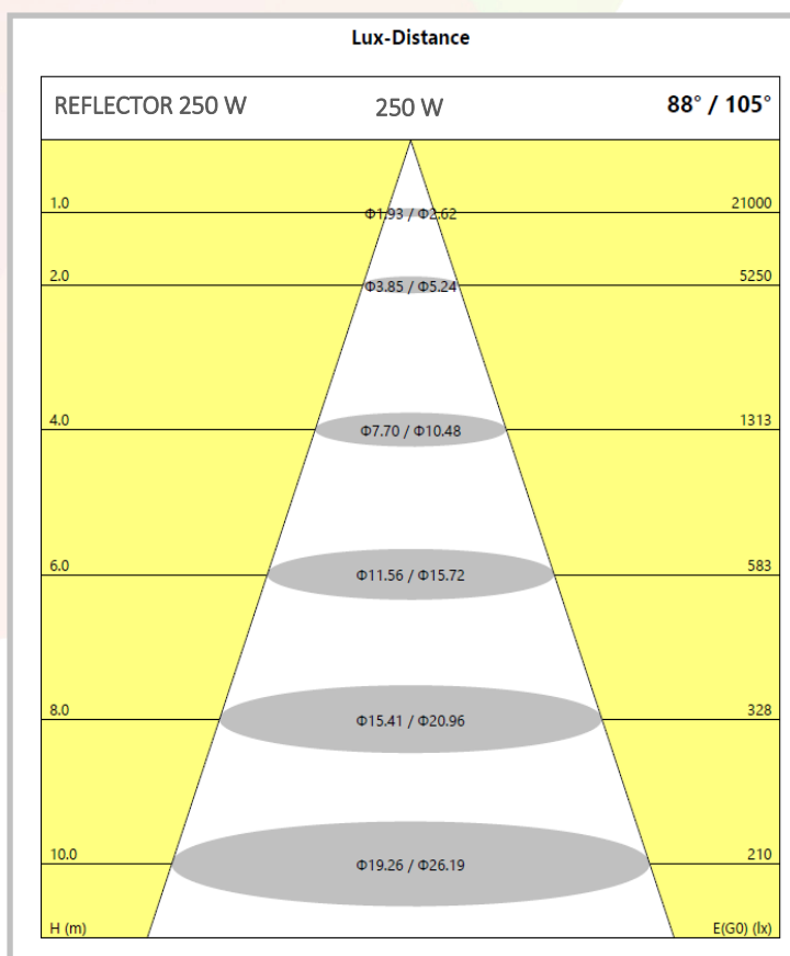
RELACION DISTANCIA-LX
