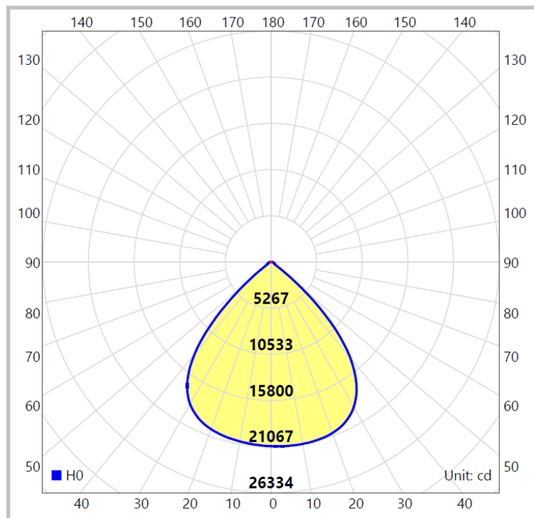
DIAGRAMA POLAR
