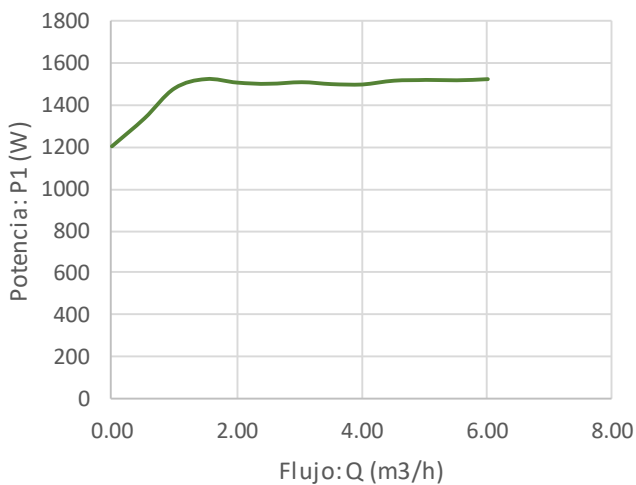
Potencia: P1 (W) vs Flujo: Q (m3/h)
