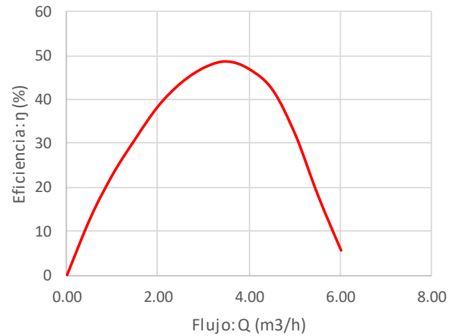
Eficiencia: \eta (%) vs Flujo: Q (m3/h)
