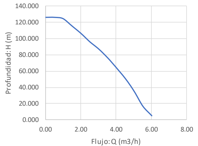
Profundidad: H (m) vs Flujo: Q (m3/h)
